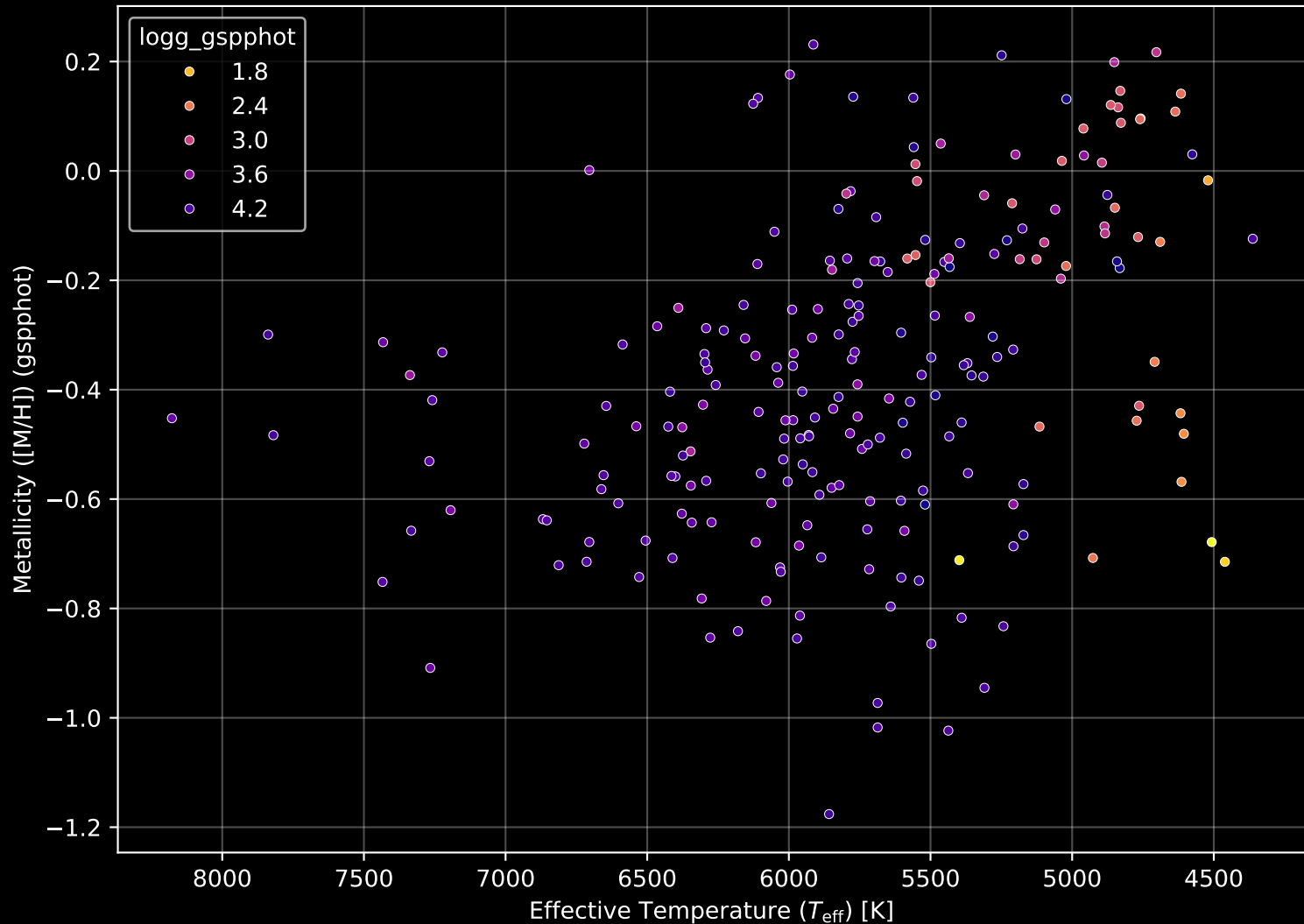
GALAH DR4 Field: [7236] Stellar Population Parameters (n= 228)
