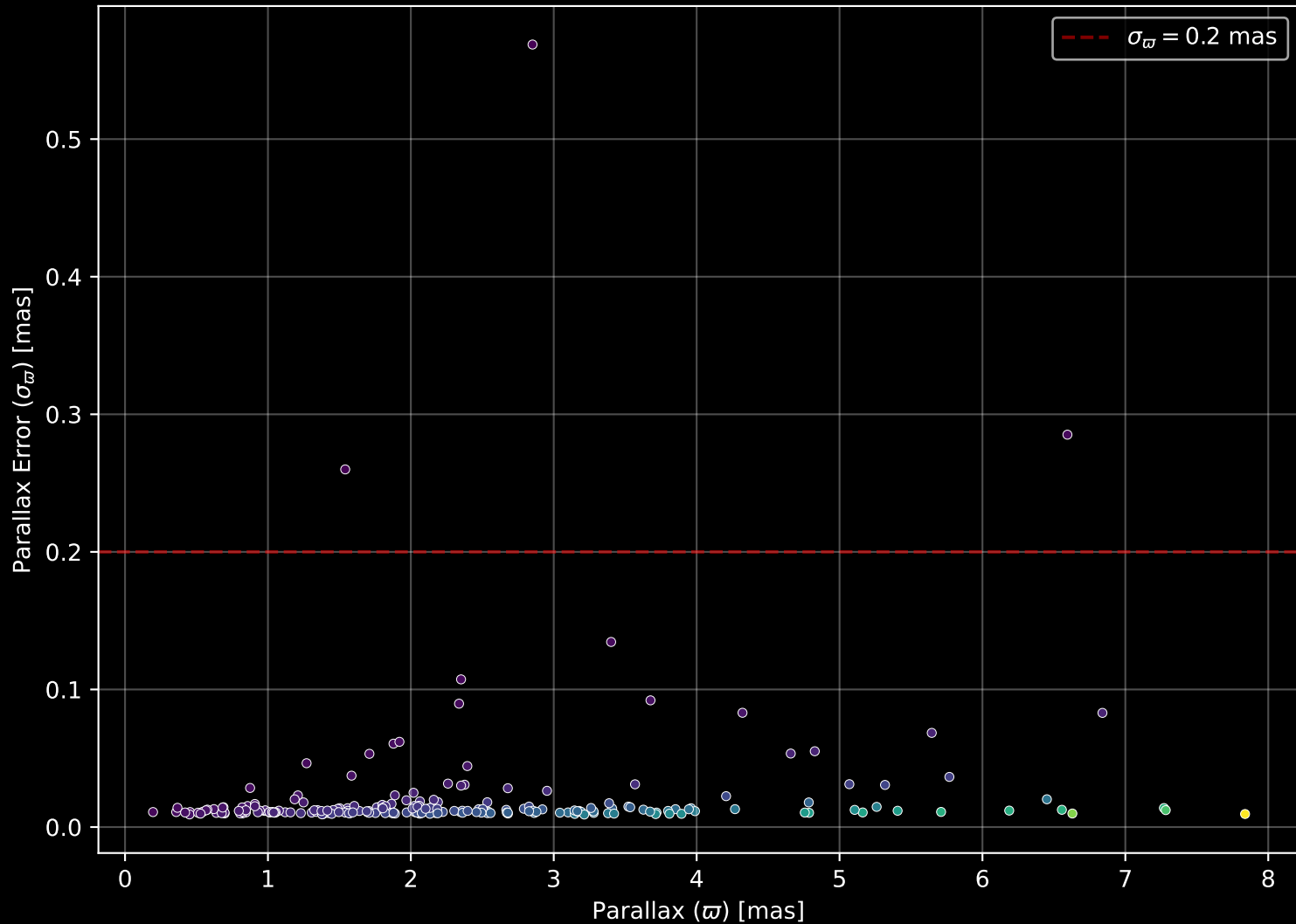
GALAH DR4 Field: [7236] Parallax Quality (n= 228)
