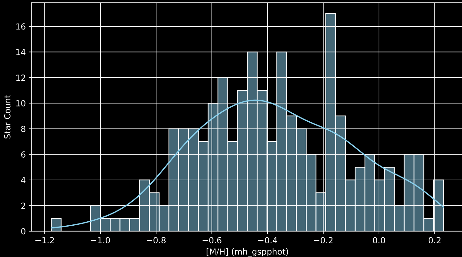
GALAH DR4 Field: [7236] [M/H] (mh_gspphot) (n= 228)
